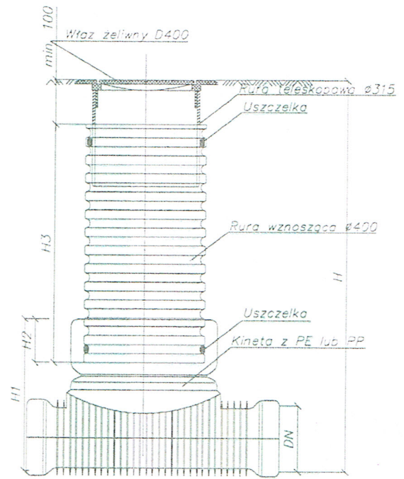
Studzienka kanalizacyjna \varnothing 400 PVC
