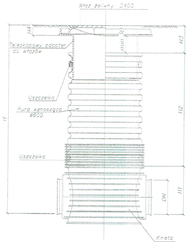
Studzienka kanalizacyjna \varnothing 600
